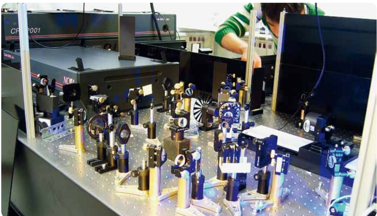
Abbildung 1: Aufbau für die Laserspektroskopie mit höchster Zeitauflösung (30 Femtosekunden)
