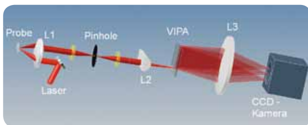
Abbildung 1: Strahlengang für die Messung der Brillouin-Streuung.
